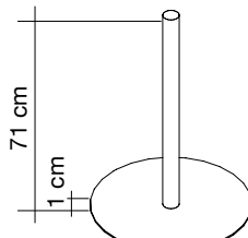
ø 50 cm 2SJ87-I
