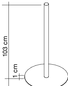
ø 50 cm 2SJ810-I
