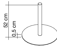
ø 50 cm 2SJ65-I
