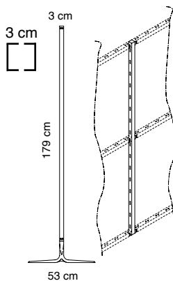
5213/BP-GA, 5213/BP-BO 2-ways up-right
