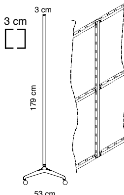
5213/BR-GA, 5213/BR-BO 2-ways up-right
