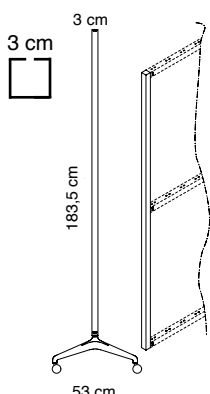
5203/BR-GA, 5203/BR-BO 1-way up-right
