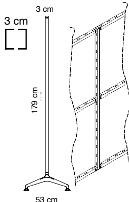
5213/B-GA, 5213/B-BO 2-ways up-right
